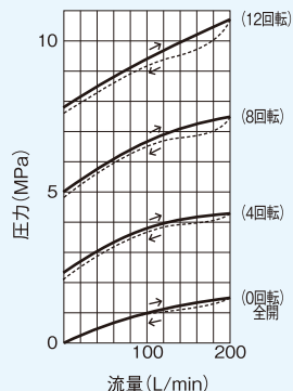
FMQ-06-P-07-21 圧力・流量特性 (粘度 32mm 2 /S)
