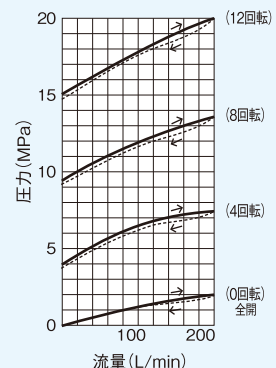
FMQ-06-P-14-21 圧力・流量特性 (粘度 32mm 2 /S)
